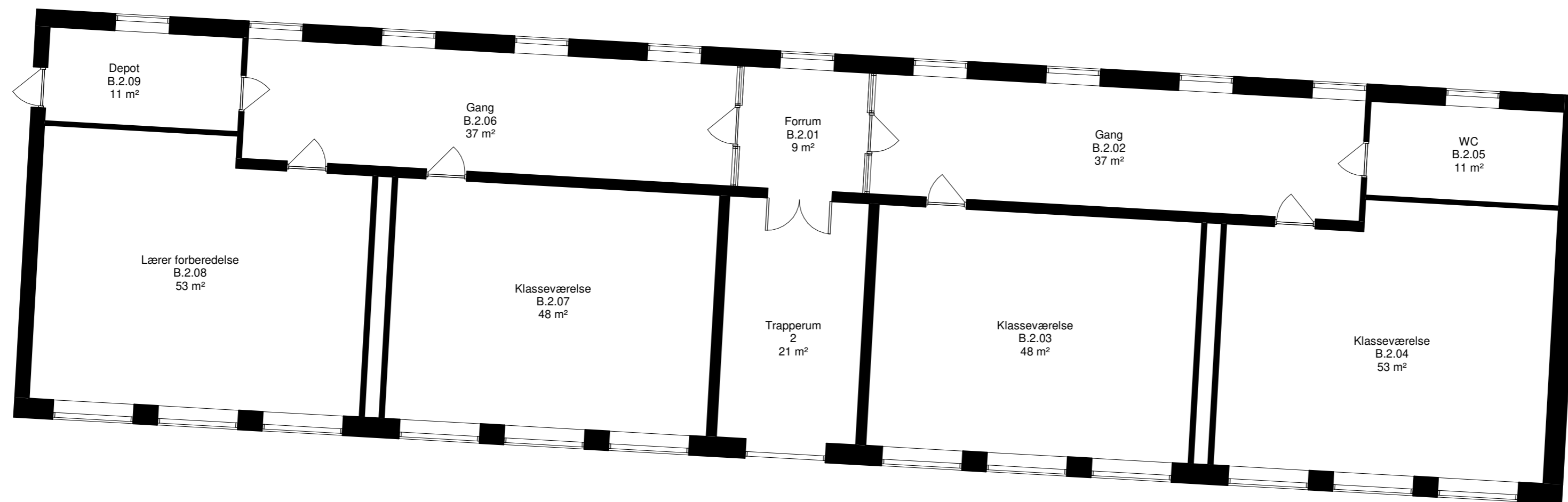
BYGNING B
